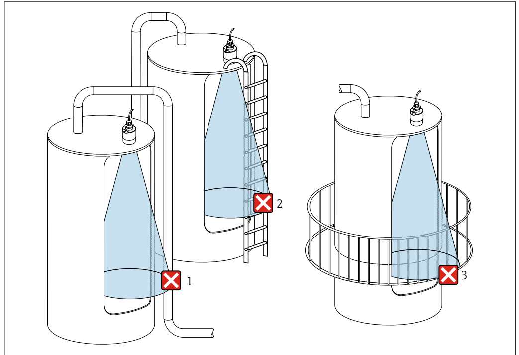
图 10 在塑料罐中测量
