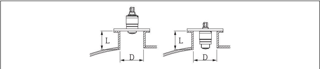
图 6 在安装短管中安装 FMR10
