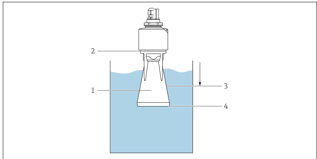
图 12 防浸没罩的功能示意图
