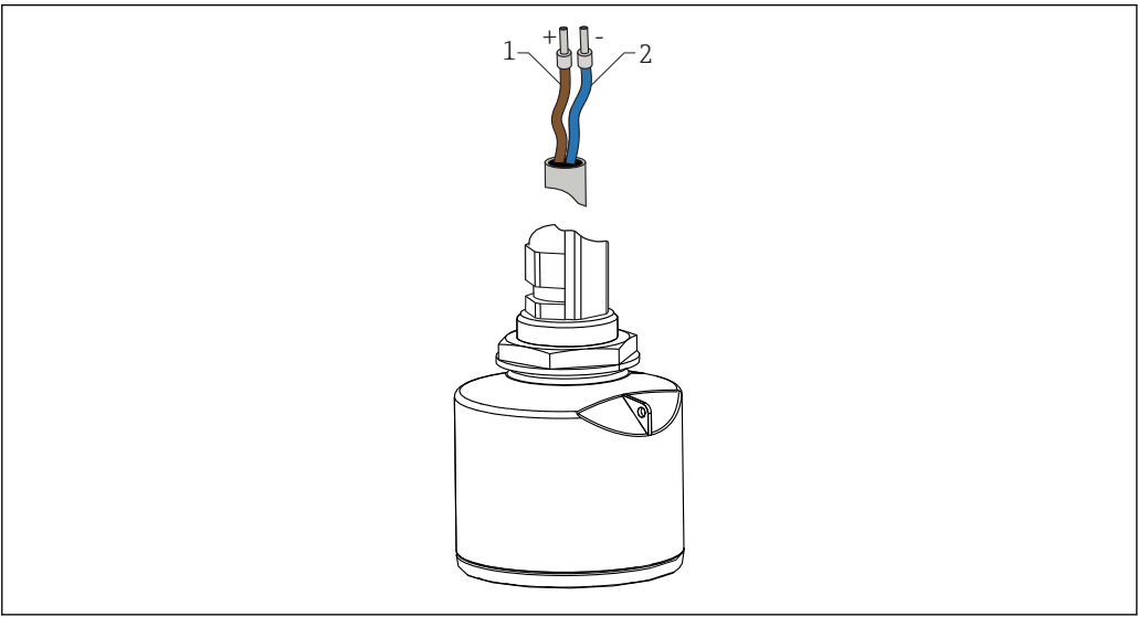
图 2 电缆分配 1 正极，棕色线 2 负极，蓝色线
