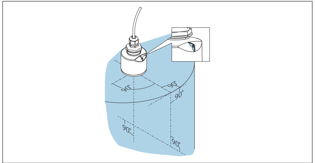
图 8 罐体中的传感器安装方向
