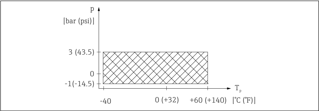
15 FMR10: 允许过程温度和过程压力范围
