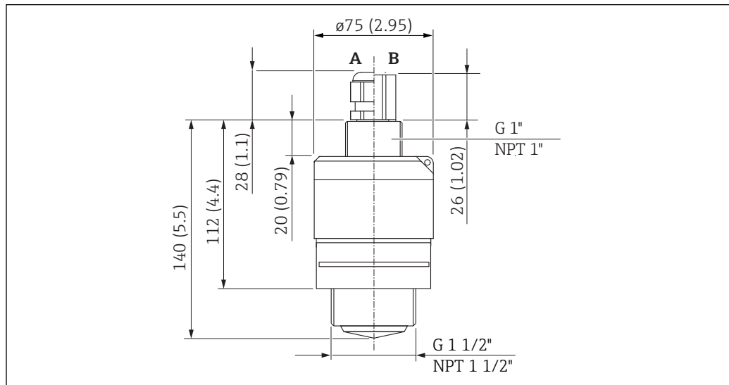
图 16 G 1-1/2" 或 MNPT 1-1/2" 螺纹过程连接的外形尺寸; 单位: mm (in)
