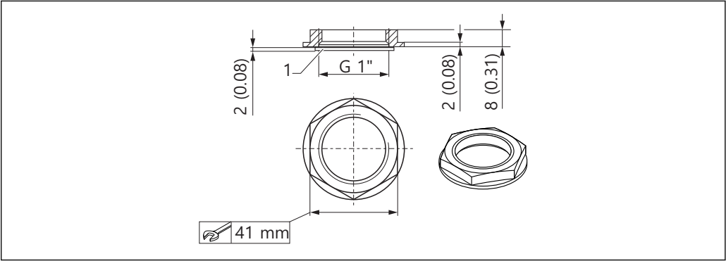
18 锁紧螺母的外形尺寸，适用于过程连接（背面）；单位：mm (in)
