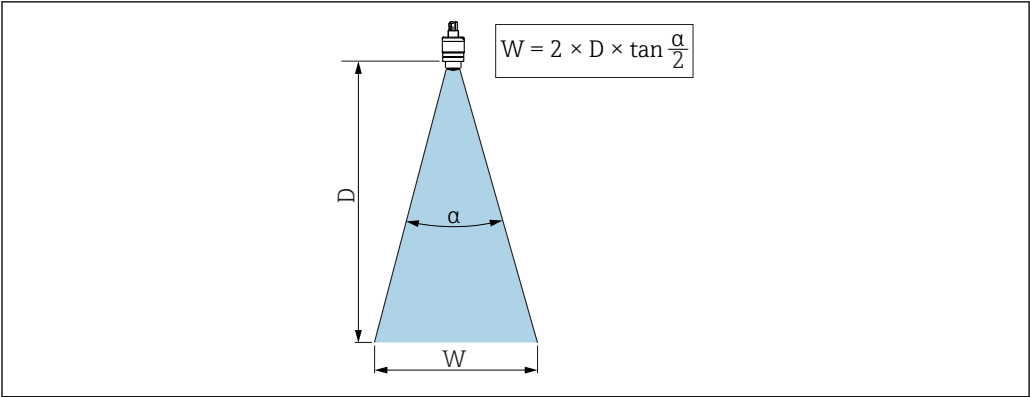
图 9 波束角 α、距离 D 和波束宽度 W 的相互关系
