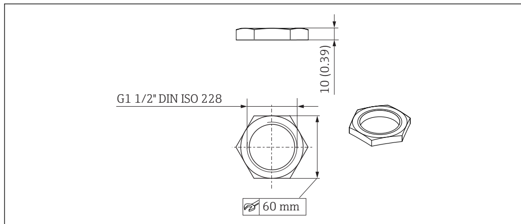
图 22 锁紧螺母的外形尺寸；单位：mm (in)
