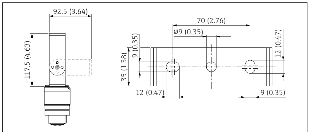
图 23 墙装支架的外形尺寸；单位：mm (in)
