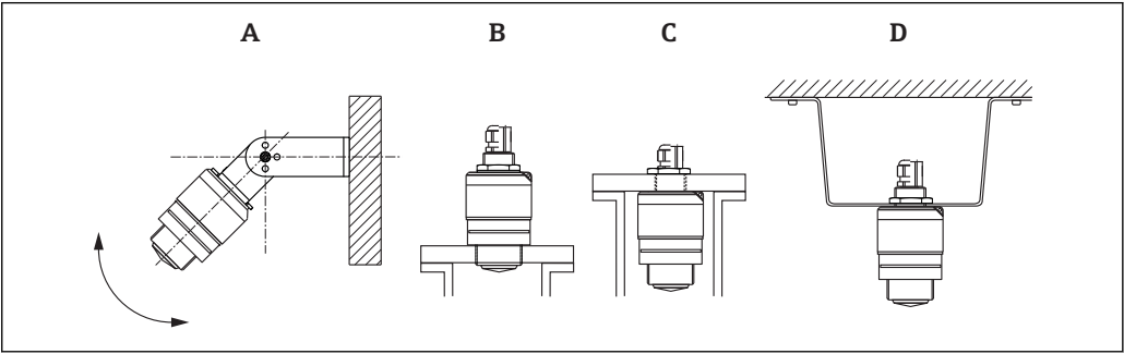
图 5 安装在墙壁上、罐顶上或安装短管中
