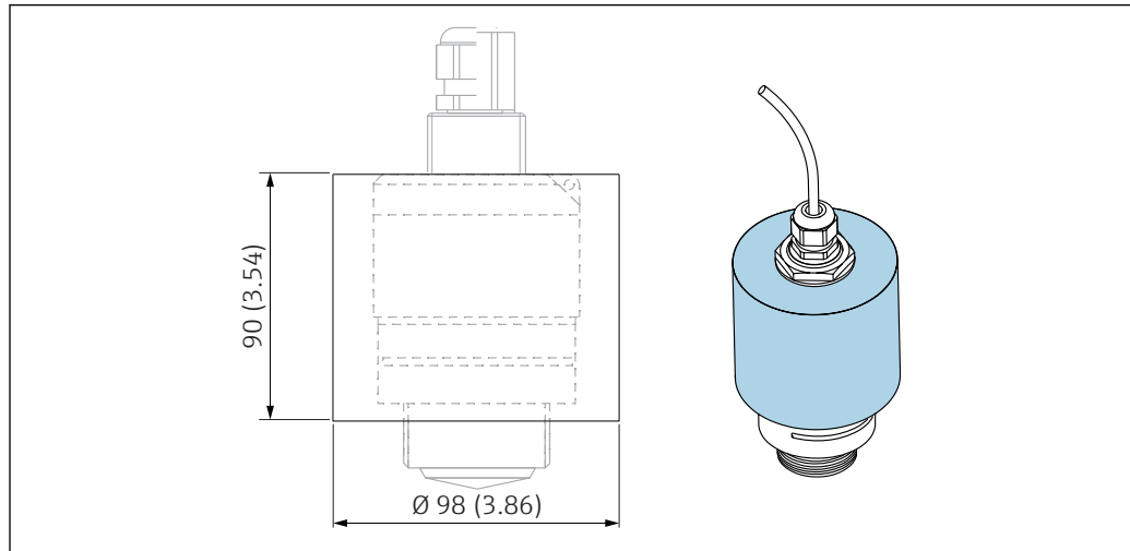
图 21 防护罩的外形尺寸；单位：mm (in)
