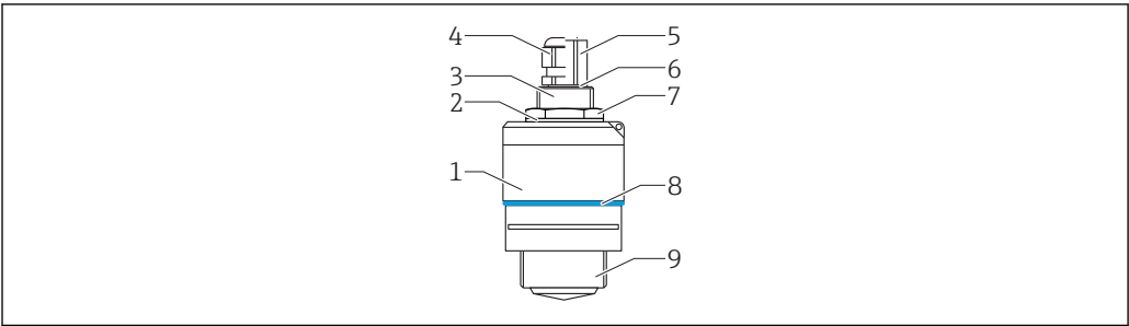
图 19 FMR10 的材质
